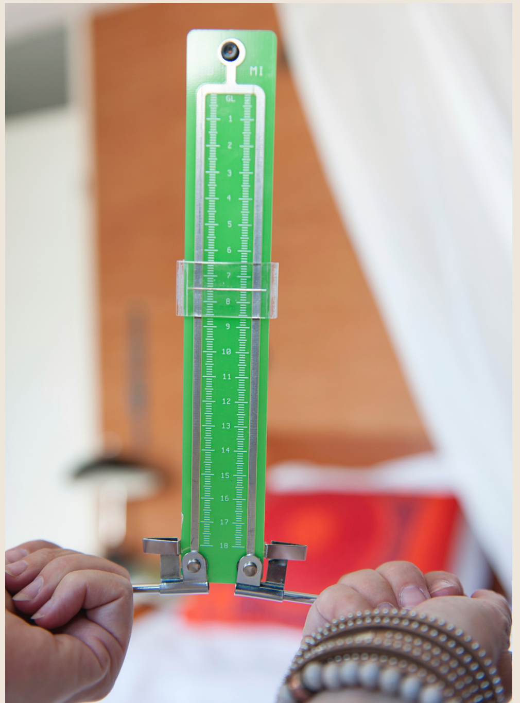
DE LECHER-ANTENNE
